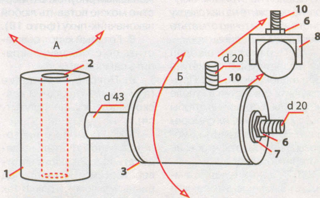
Рис. 2 Сцепное устройство в сборе А и Б — направления степеней свободы, используемые при поворотах и неровностях дороги
