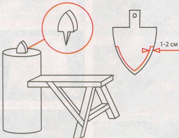
Рис. 1 Отбивочный станок
