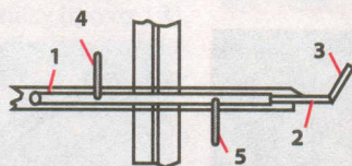
Рис. 3 Засов
